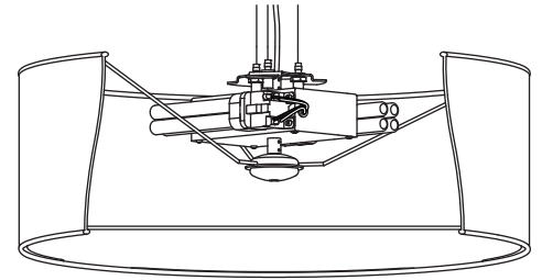
VUE COUPÉE OPTION FLUORESCENT
