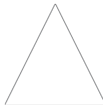
gl.LINE_LOOP
