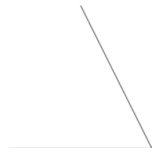
gl.LINE_SET
